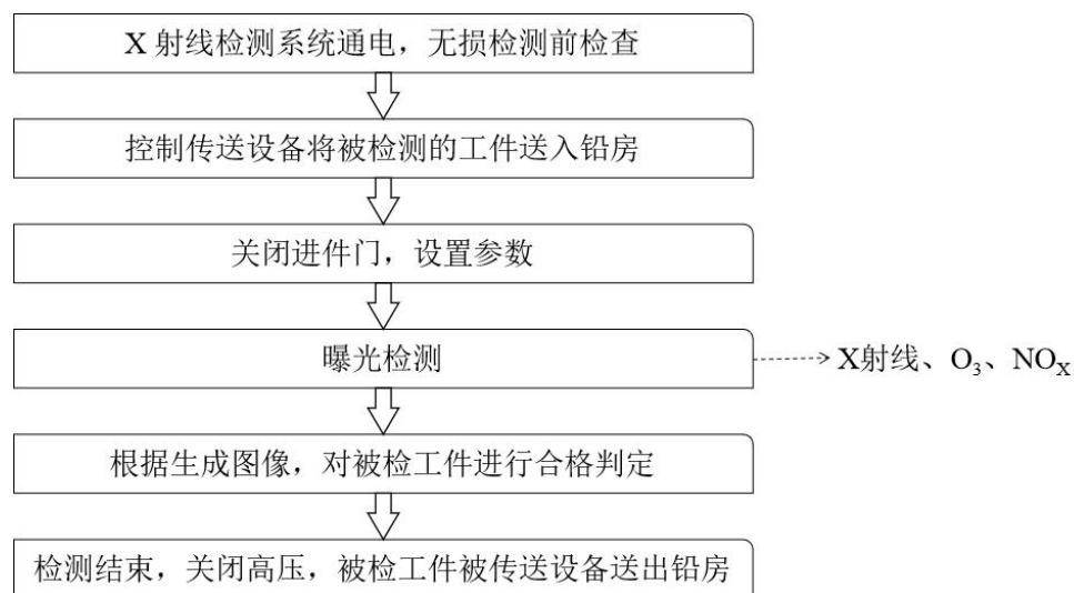
图 9-6 本项目 ZXFC450 型智能型 X 射线 DR 检测系统工艺流程及产污环节分析示意图
