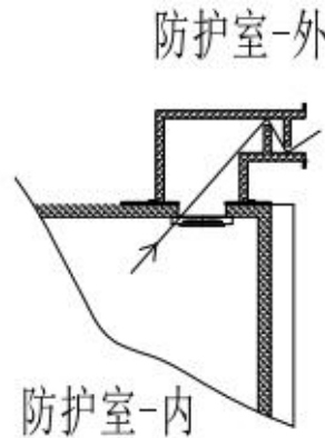
图 11-2 迷道设计电缆口防护罩结构散射示意图
