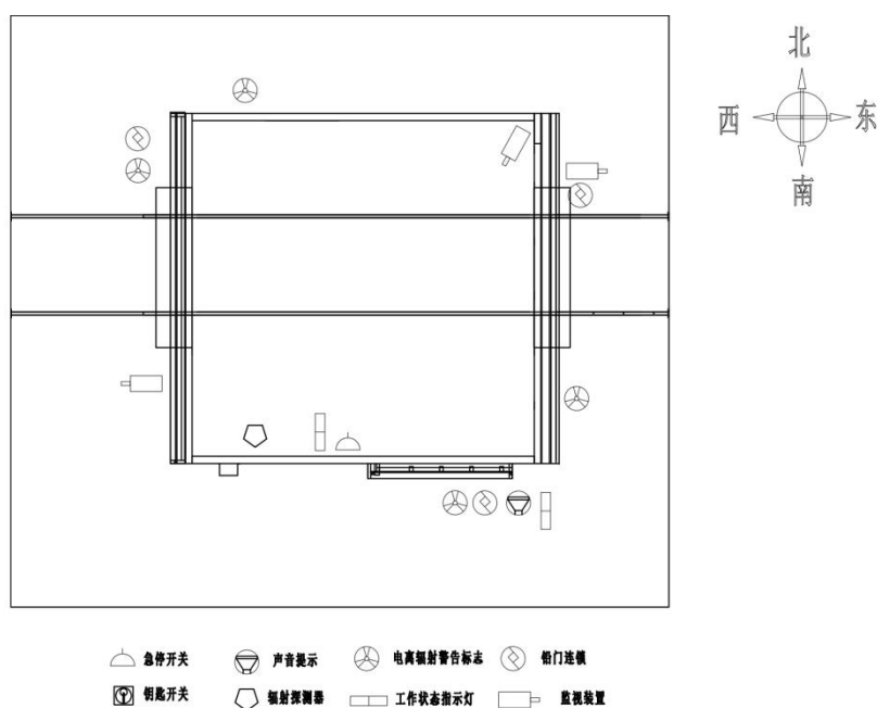
图 10-5 本项目 XYG22508/3 型 X 射线数字检测成像系统辐射安全与防护措施布置图
