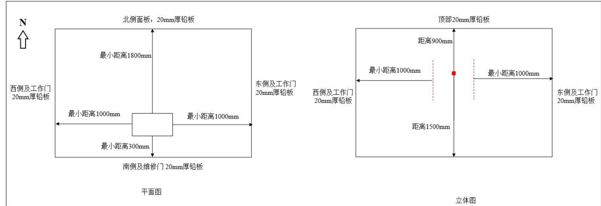
图 10-3 本项目 XYG22508/3 型 X 射线数字检测成像系统铅房屏蔽参数
