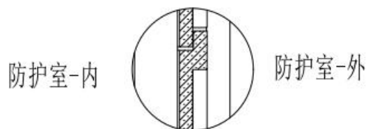
图 11-4 防护门搭接设计示意图
