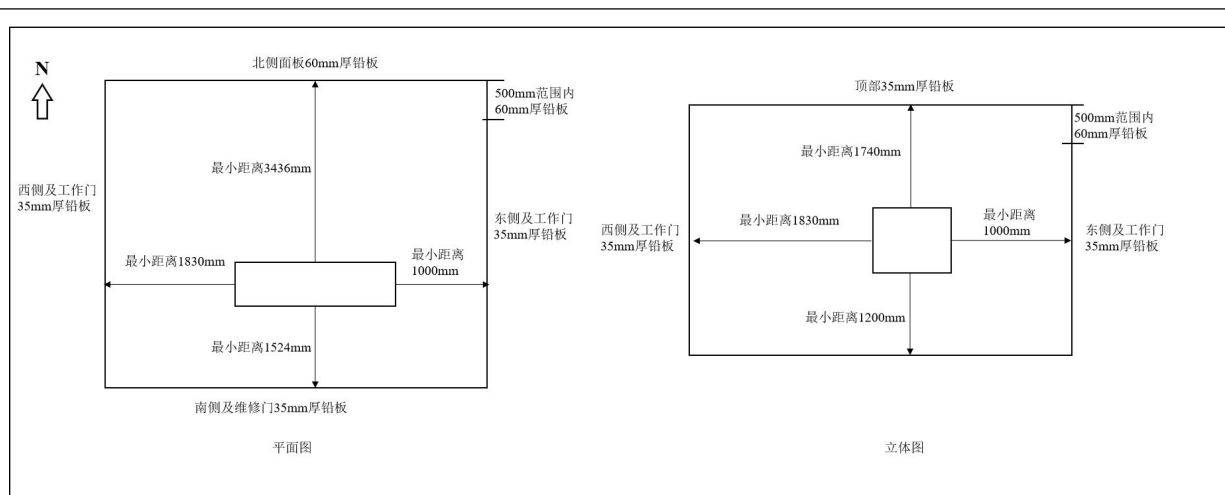
图 10-4 ZXFC 450 型智能型 X 射线 DR 检测系统铅房屏蔽参数
