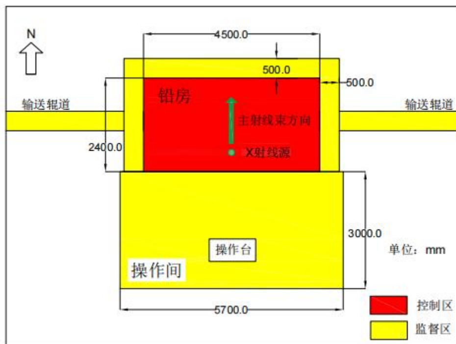
图 10-1 本项目 XYG22508/3 型 X 射线数字检测成像系统监督区及控制区示意图
