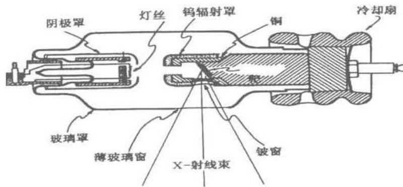
图 9-4 典型的 X 射线管结构图
