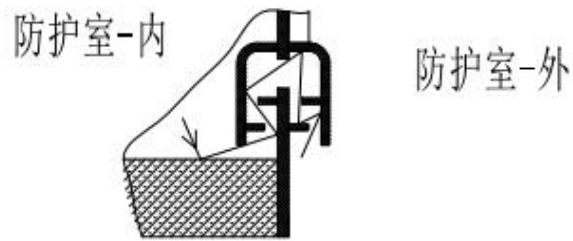
图 11-2 迷道设计电缆口防护罩结构散射示意图
