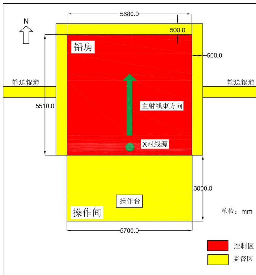
图 10-2 本项目 ZXF C 450 型智能型 X 射线 DR 检测系统监督区及控制区示意图
