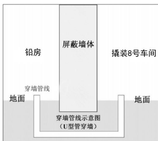
图 11-1 埋地设计电缆口防护罩结构散射示意图
