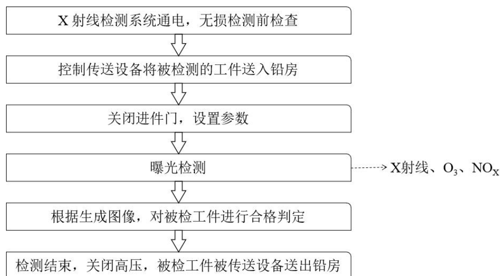
图 9-5 本项目 XYG22508/3 型 X 射线数字检测成像系统工艺流程及产污环节分析示意图
